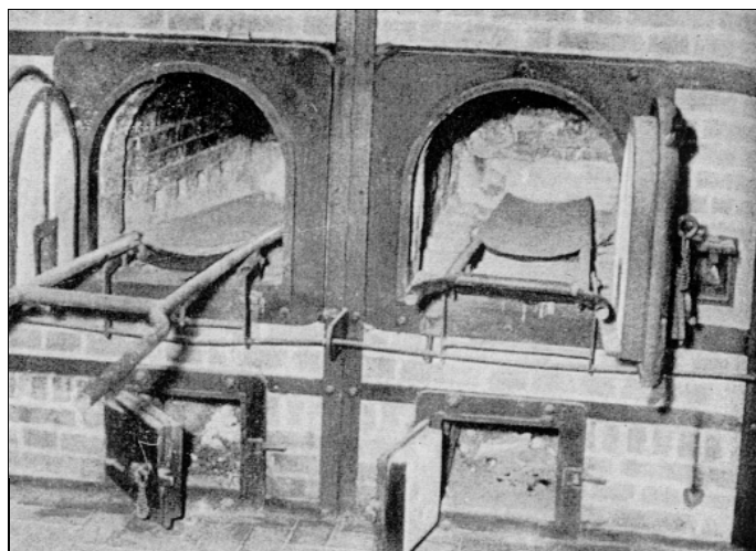
Abb. 1: Typischer Topf-Doppelmuffel-Einäscherungs-ofen in der Kriegsversion. Obere Schließknebel am Türrahmen fehlen. Vermutlich einzige veröffentlichte Innenaufnahme des Birkenauer Krematoriums, welches vier solcher Anlagen hatte. (VffG 2/98, S. 124)
